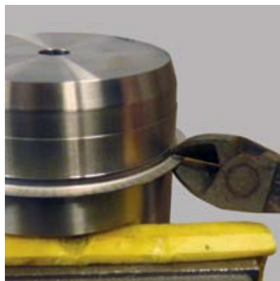
Вал с установленной втулкой/ Shaft with attached WSH R
