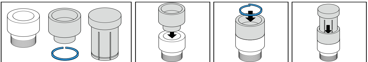
Einbau Führungselemente | Yataklama elemanları montajı | Instalacja elementów prowadzących | Монтаж направляющих элементов
