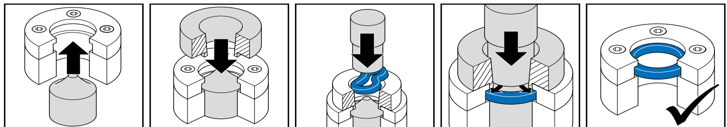
1B. Einbau mit Pusher, Konushülse und Gegenhalter | İtici, konik kol ve tutucu ile montaj | Instalacja za pomocą popychacza, rękawa stożkowego, blokad | Установка с помощью толкателя, конусной втулки и контрупора
